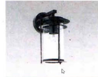
96241 VALDEO wall luminaire; galvanized steel, copper-antique / glass, clear Wandleuchte; Stahl verzinkt, kupferfarben-antik / Glas, klar applique; acier galvanisé, cuivré / verre, clair L 165, H 275, A 200
